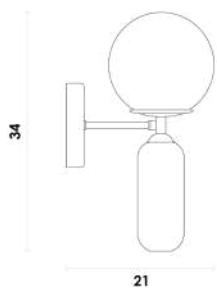
Arandela Metal / Vidro E27 1X25W
