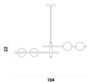
Pendente Metal / Vidro G9 4X25W
