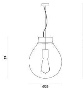
Pendente Vidro / Metal E14 1X40W
